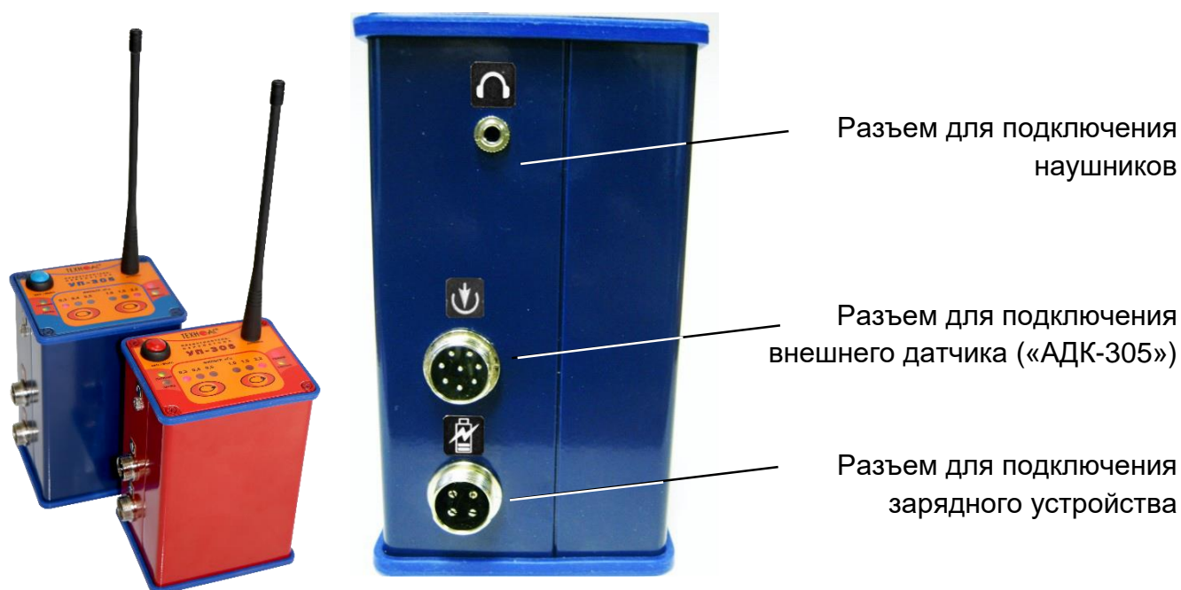
Рисунок 3 Предусилители-передатчики УП-305 «синего» и «красного» каналов (слева) и расположение разъемов на корпусе
